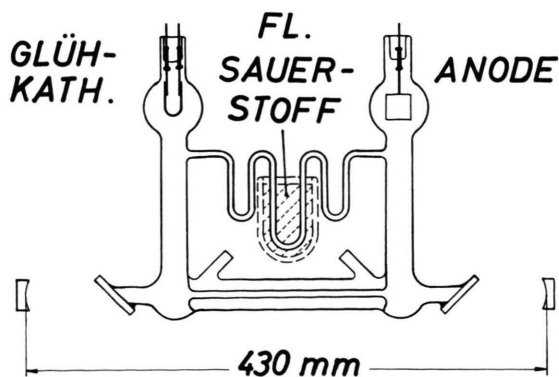
Abb. 1. Xenon-Ionen-Laser, schematisch.
